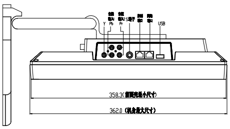
左侧视图
