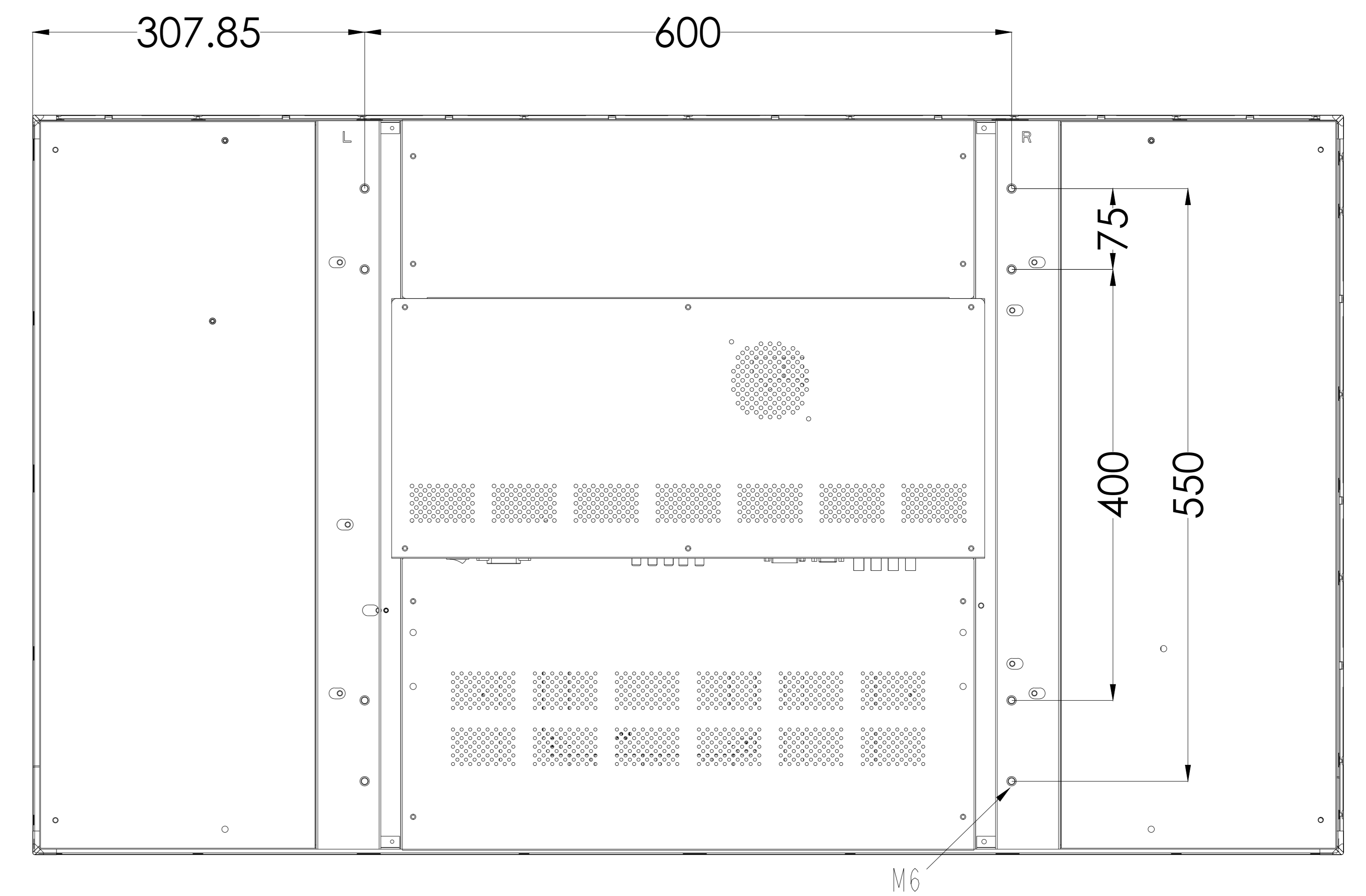
后视图
